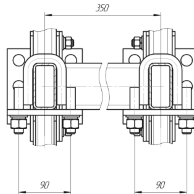
Б-Б (1:2,5) (2 места)
